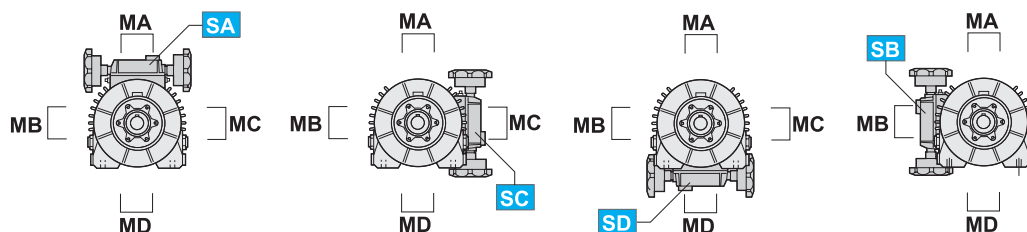
Posizione morsettiere e scatola di comando
